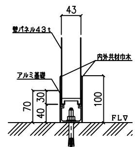
《 床断面図 》
