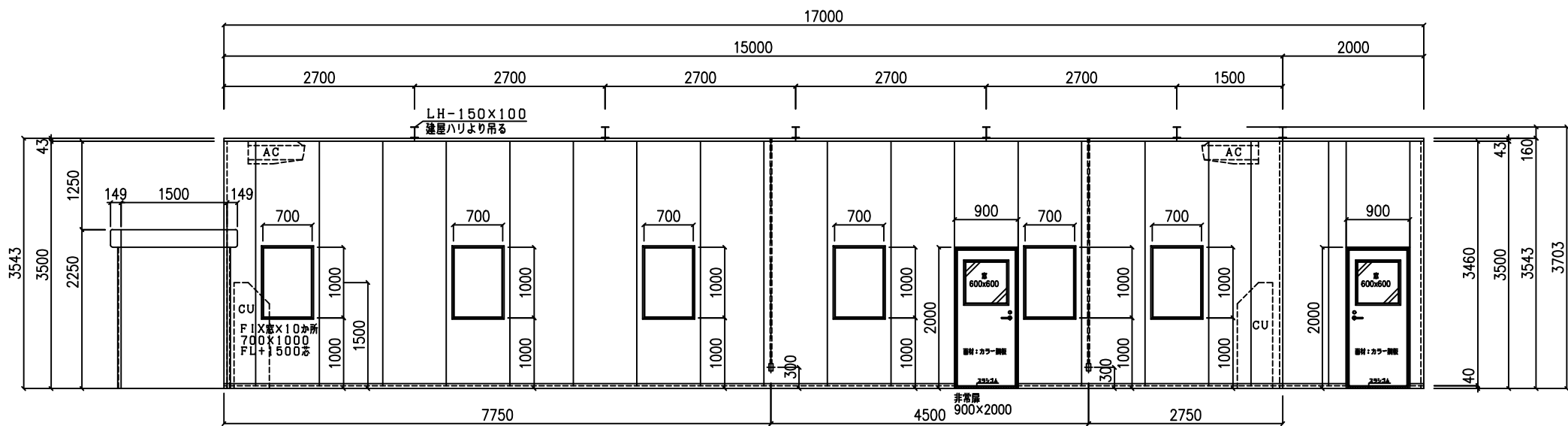
《 ア-立面図 》
