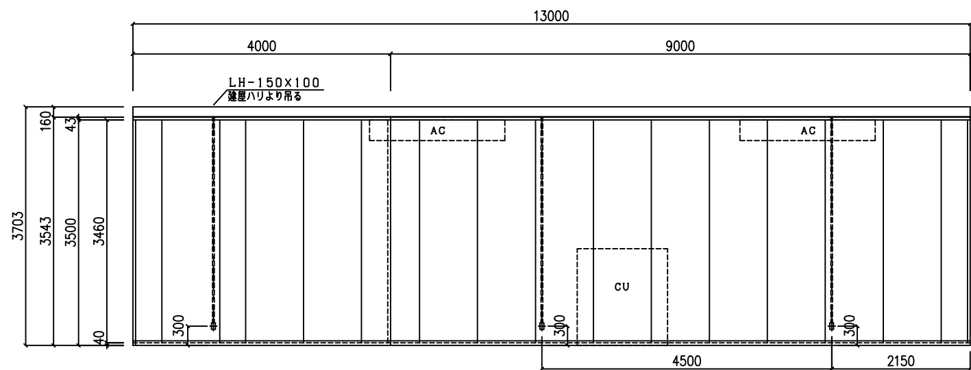
《 II-立面図 》
