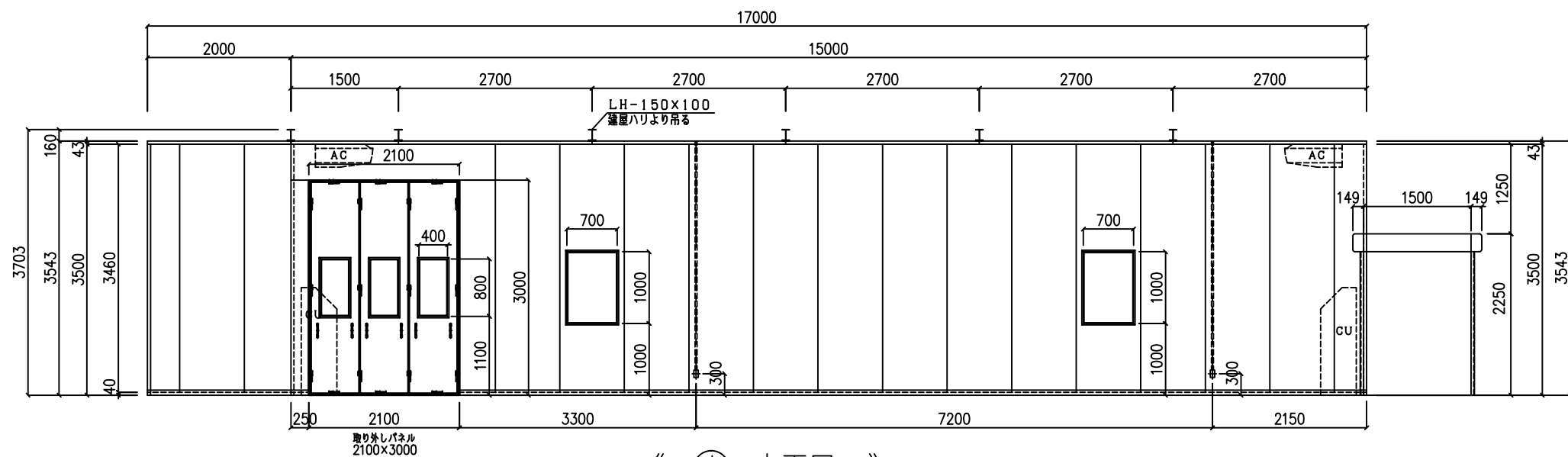
《 ウ-立面図 》
