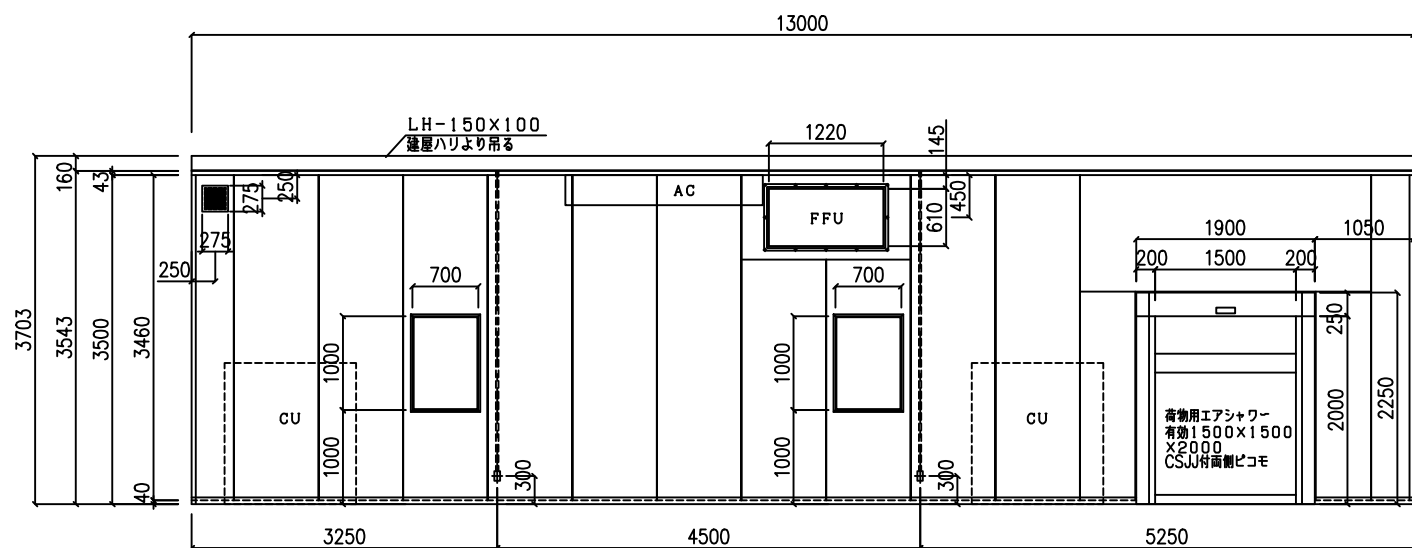
《 イ-立面図 》
